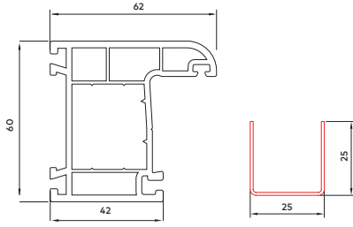
60 mm Çerçivə Profili
