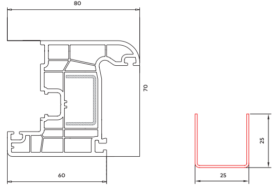
70 mm Qanad Profili
