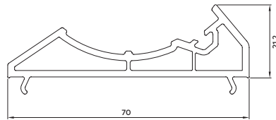
Köşe Dönüş Profili
