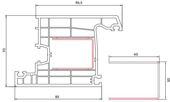
70 mm İç Açılan Qapı Profili
