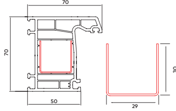
70 mm Çerçeve Profili
