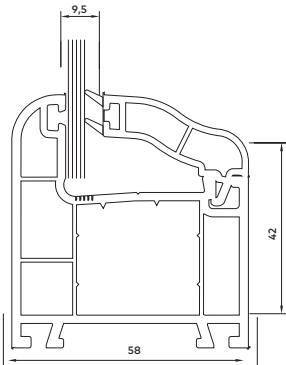
58 mm Tək Paket Çita
