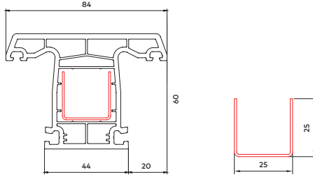
60 mm Orta Bağlantı Profili
