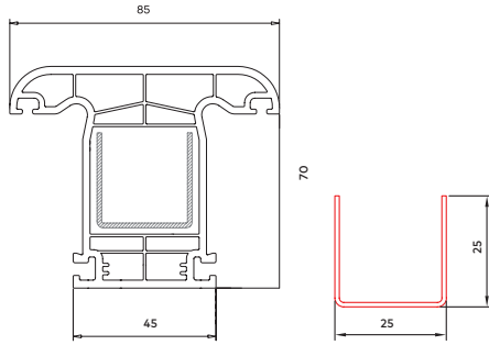
70 mm Orta Bağlantı Profili
