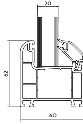
60 mm Cüt Paket Çita
