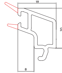
60 mm Cüt Paket Çita
