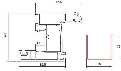
60 mm Qanad Profili
