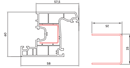
60 mm Qanad Profili
