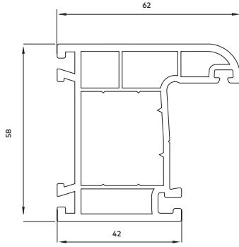
58 mm Çerçeve Profili
