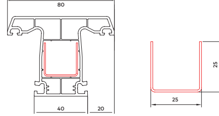
60 mm Orta Bağlantı Profili
