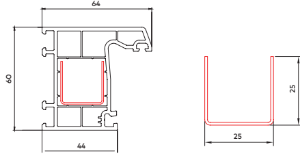
60 mm Çerçeve Profili
