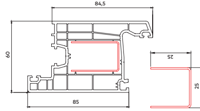
60 mm Qapı Qanadı Profili
