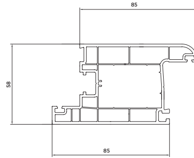
58 mm Qapı Qanadı Profili
