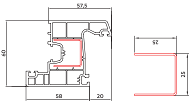
60 mm Qanad Profili
