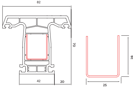
70 mm Orta Bağlantı Profili
