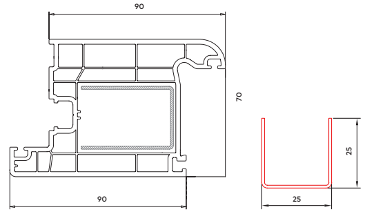
70 mm Qapı Qanadı Profili
