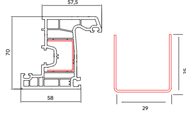
70 mm Qanad Profili
