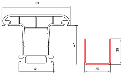
60 mm Qapı Qanadı Profili
