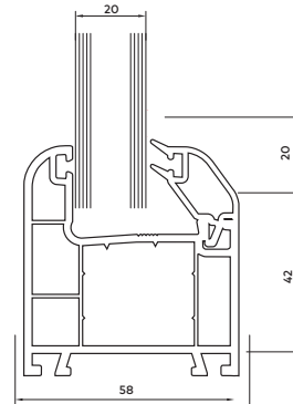
58 mm Cüt Paket Çita
