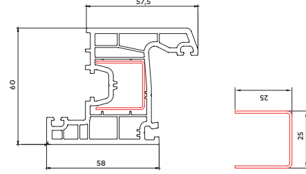
60 mm Qanad Profili
