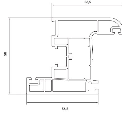
58 mm Qanad Profili
