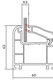
60 mm Tək Paket Çita
