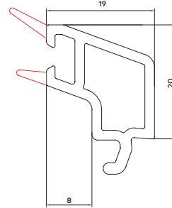
60 mm Cüt Paket Çita
