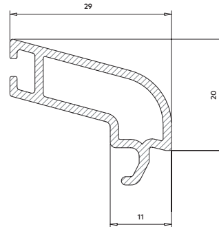
70 mm Cüt Paket Çita
