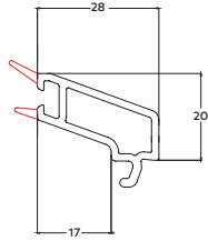
70 mm Cüt Paket Çita
