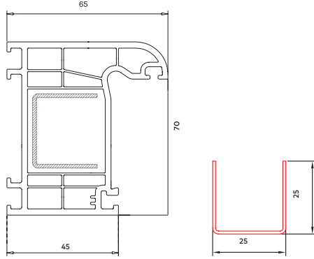
70 mm Çerçive Profili
