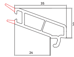
60 mm Tək Paket Çita
