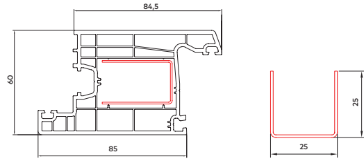
60 mm Qapı Qanadı Profili
