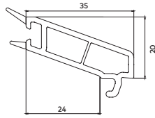
60 mm Tək Paket Çita
