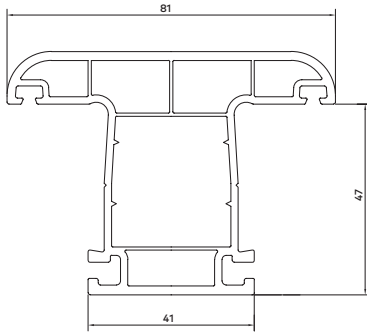
58 mm Orta Bağlantı Profili
