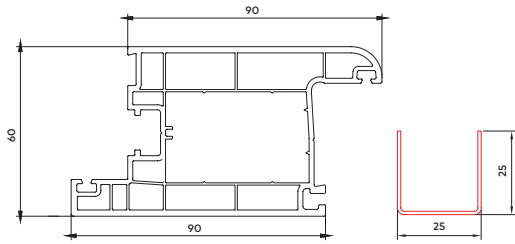
60 mm Qapı Qanadı Profili
