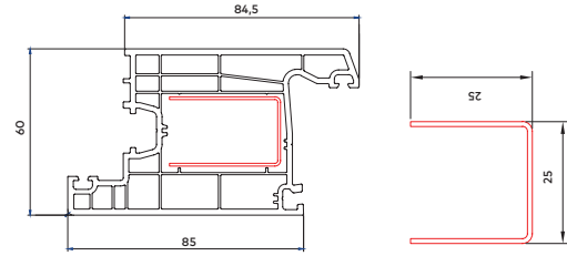
60 mm Qapı Qanad Profili
