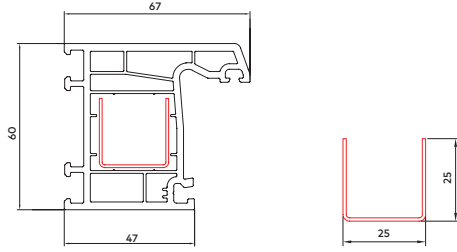
60 mm Çerçive Profili
